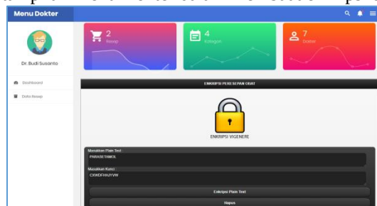
Gambar 5. Enkripsi Data Obat
