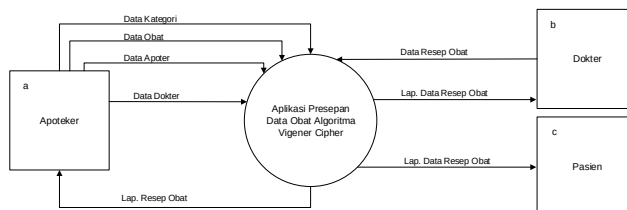
Gambar 3. Kontek Diagram Sistem
